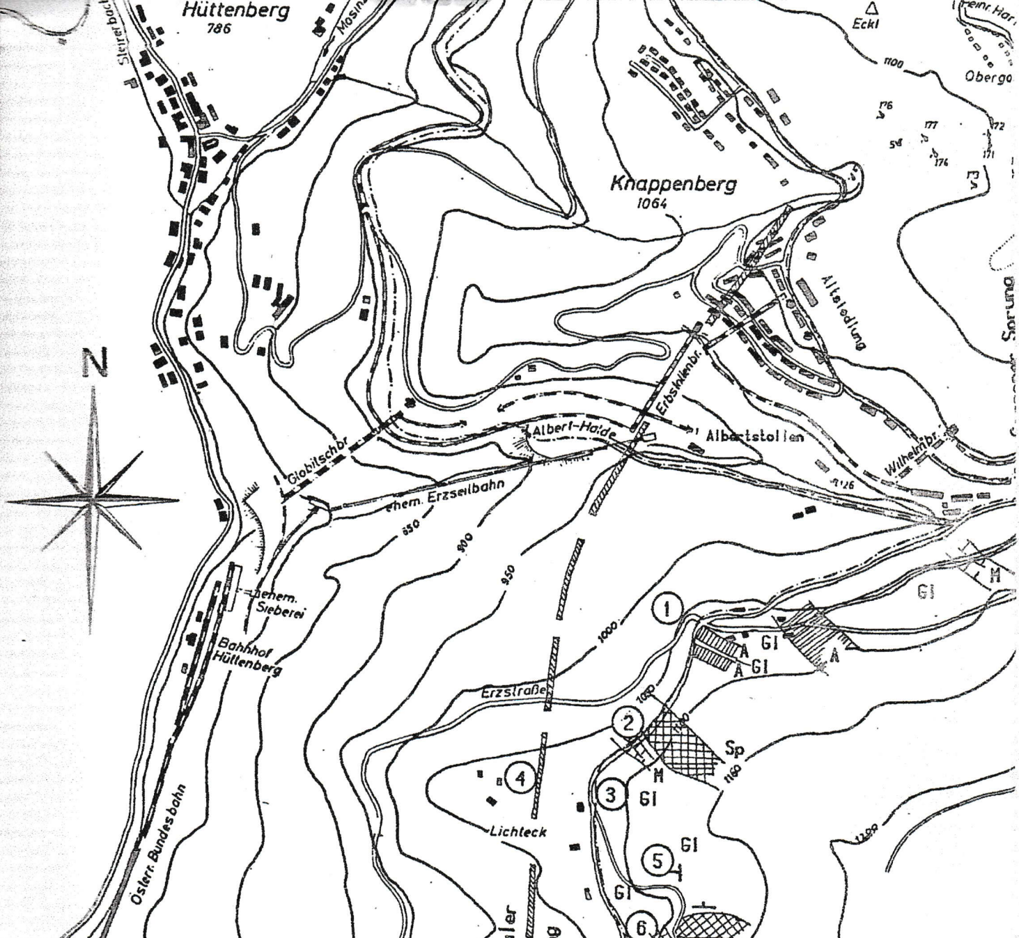
E. CLAR, 1983 : PETROGRAPHISCH- GEOLOGISCHE EXKURSION UM DEN PLANKENKEGEL BEI HÜTTENBERG Kartenskizze 1 : 10.000
